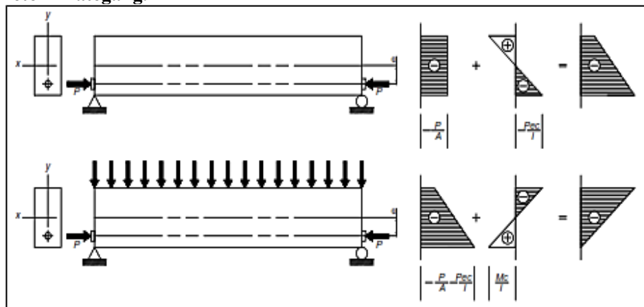
Gambar 2. (a) Tendon Eksentris, hanya prategang tanpa beban sendiri. (b) Tendon Eksentris, prategang ditambahkan beban sendiri.
