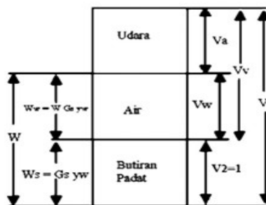
Gambar 1. Tiga fase elemen tanah.
