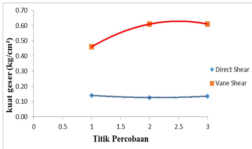
Gambar 5. Perbandingan Uji Geser Langsung Dan Uji Geser Baling Kedalaman
