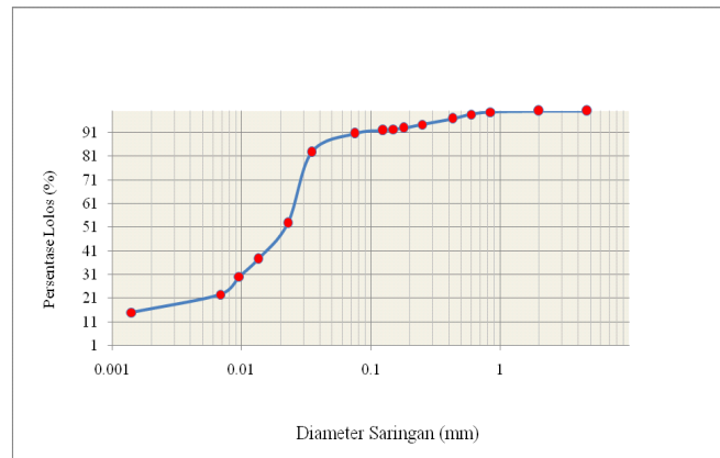
Gambar 1. Grafik Diameter Butiran Tanah
