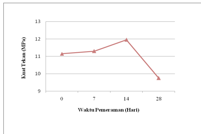
Gambar 3. Hubungan Antara Nilai Kuat Tekan Paving Block Pasca Pembakaran dengan Jangka Waktu Pemeraman
