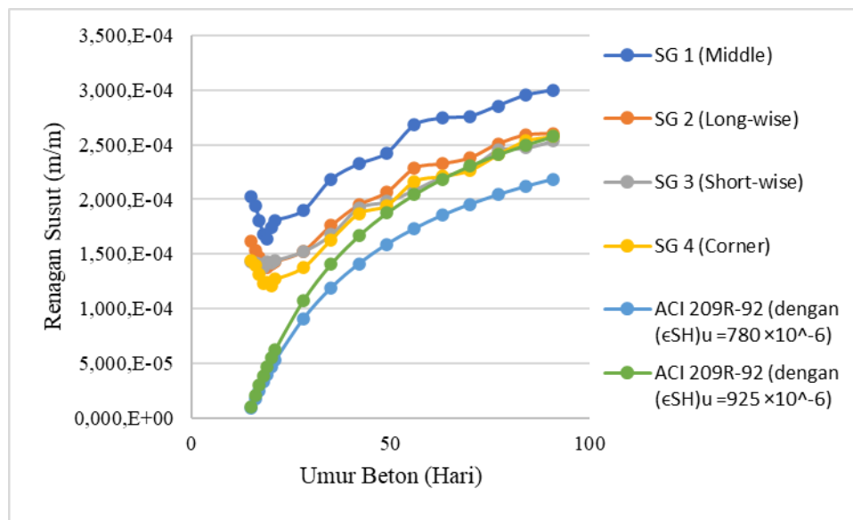
Gambar 4. Perbandingan Regangan yang Diteliti dengan ACI 209R-92
