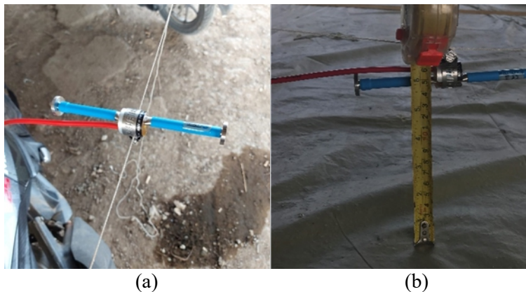
Gambar 3. Pemasangan alat VWSG (a) pengikatan kawat dengan tali (b) pengukuran ketinggian alat.
