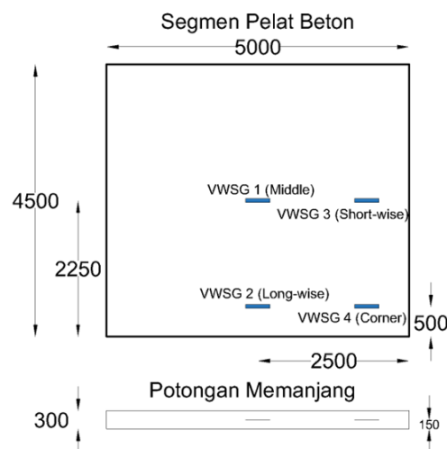
Gambar 1. Skema penempatan VWSG pada segmen pelat beton.
