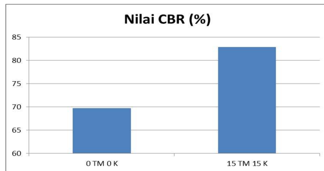
Gambar 3. Perbandingan Hasil Uji CBR
