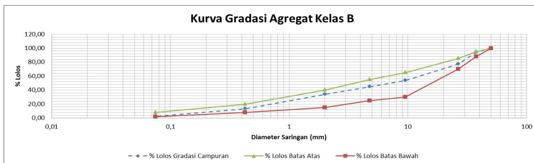
Gambar 2. Grafik analisa saringan
