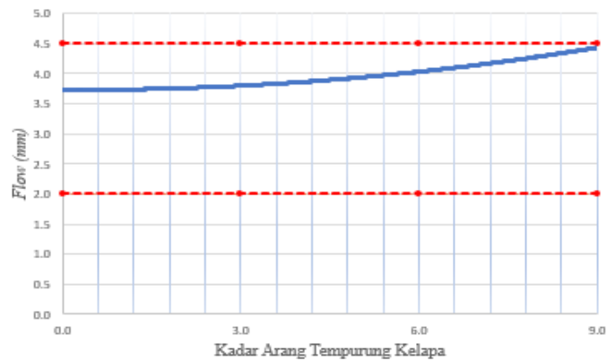
Gambar 3. Grafik Flow Terhadap Arang Tempurung Kelapa.
