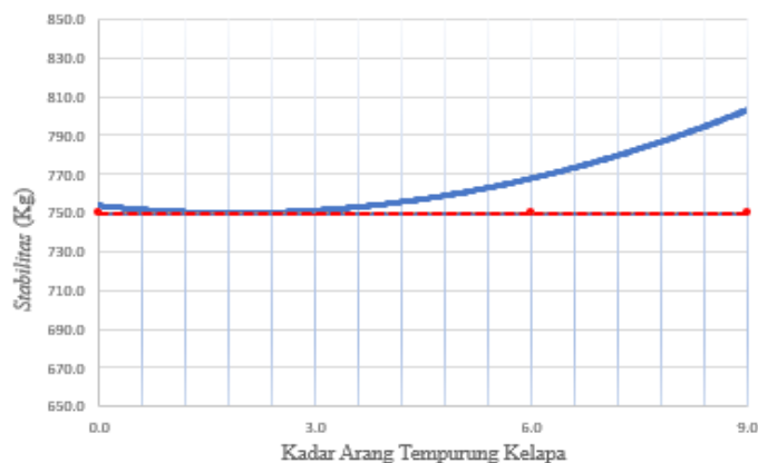
Gambar 2. Grafik Stabilitas Terhadap Arang Tempurung Kelapa.
