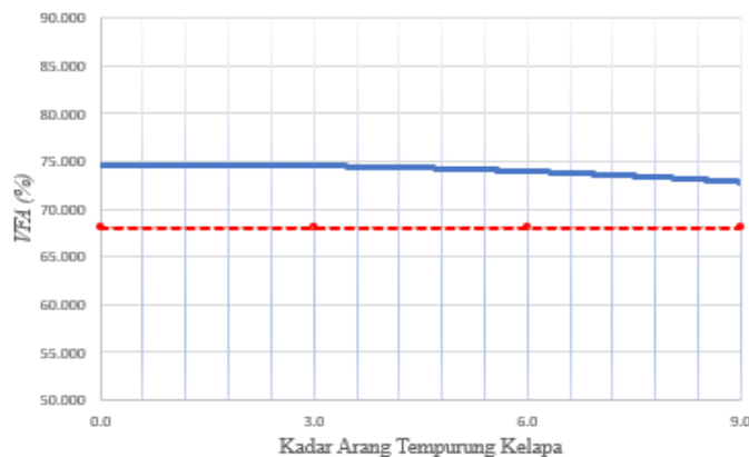
Gambar 6. Grafik VFA Terhadap Arang Tempurung Kelapa.
