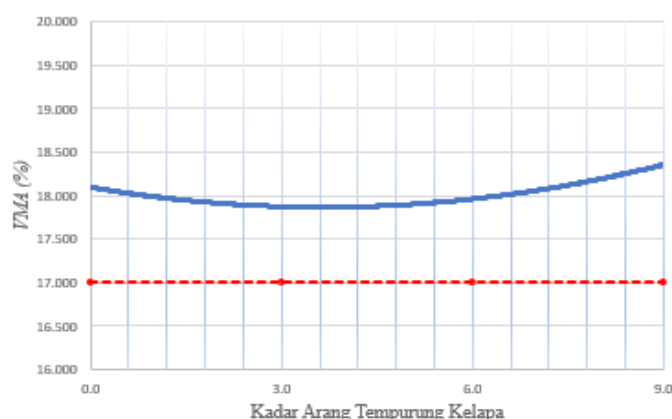
Gambar 5. Grafik VMA Terhadap Arang Tempurung Kelapa.
