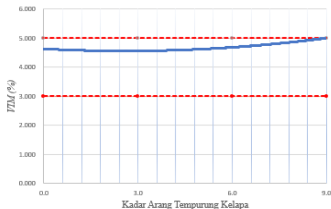
Gambar 4. Grafik VIM Terhadap Arang Tempurung Kelapa.
