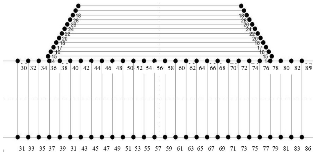
Gambar 3. Desain perbaikan tanah menggunakan metode preloading dan PVD dengan jarak 8 m
