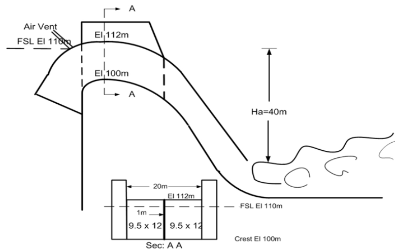
Gambar 1. Siphon Spillway
