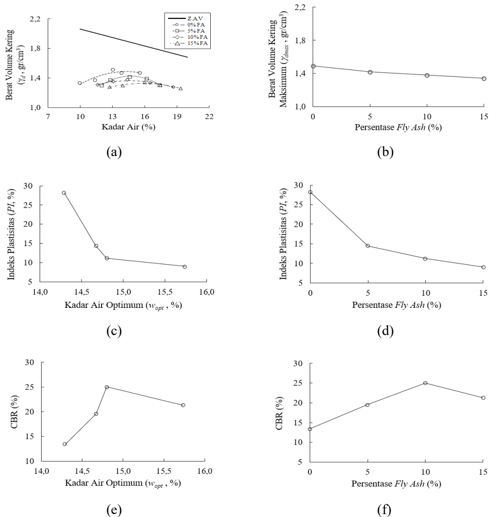
Gambar 5. Grafik pengujian campuran tanah dan fly ash variasi pemeraman 7 hari pada suhu pemeraman 40°C.
