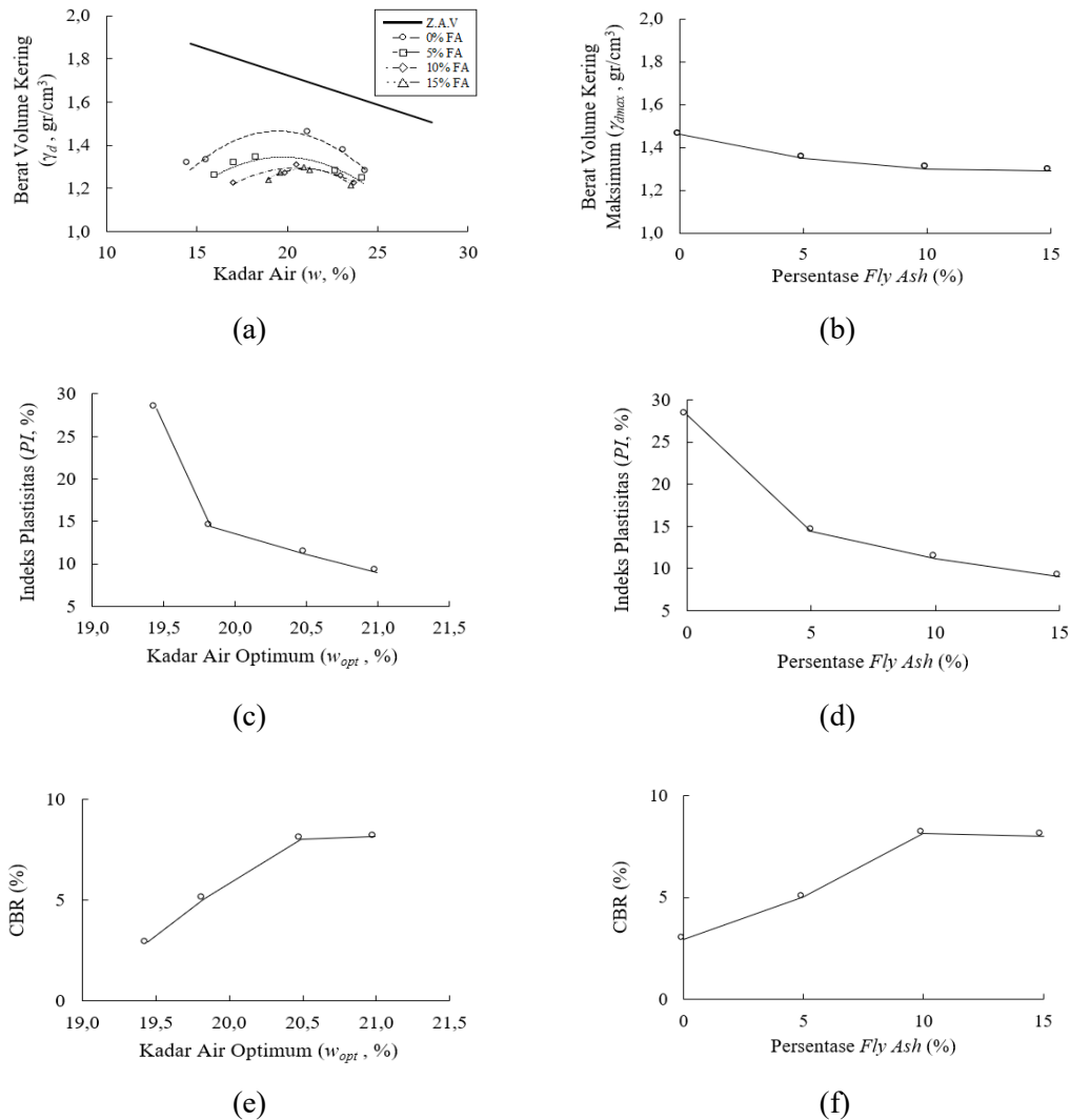
Gambar 4. Grafik pengujian campuran tanah dan fly ash tanpa pemeraman.
