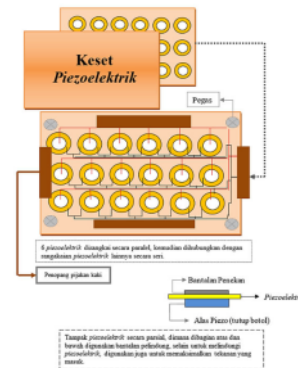
Gambar 3.3. Desain Keset Piezoelektrik.
