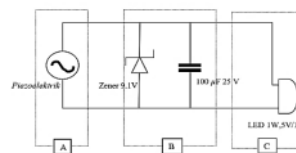
Gambar 3.4. Diagram desain keset piezoelektrik.
