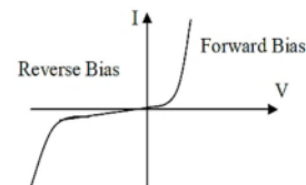
Gambar 2.8. Karakteristik dioda zener. [19]
