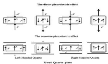
Gambar 2.1. Efek langsung ( direct ) dan terbalik ( converse ) Piezoelektrik. [18]
