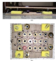
Gambar 4.2. Tampak samping (a) dan atas (b) keset piezoelektrik .
