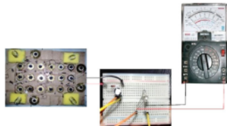
Gambar 4.1. Pengukuran rangkaian Piezoelektrik dengan multimeter.
