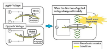
Gambar 2.2 Prinsip kerja piezoelektrik (Sumber: www.manorshi.com ).
