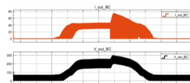
Gambar 4.4. Profil tegangan dan arus output boost converter hasil simulasi.
