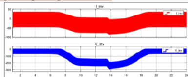
Gambar 4.5. Profil tegangan output inverter (garis biru) dan profil arus output inverter (garis merah) hasil simulasi.
