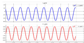
Gambar 4.10. Profil arus grid (biru) I_{grid} dan tegangan grid (merah) V_{grid} hasil simulasi dalam siklus 0,2 detik.
