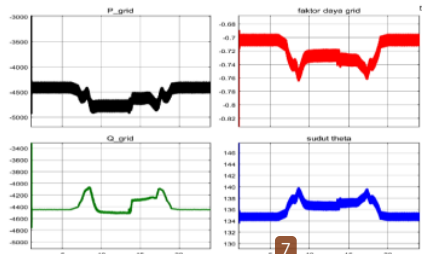
Gambar 4.11. Profil output grid: daya aktif P, daya reaktif Q, faktor daya \cos \theta dan sudut \theta .
