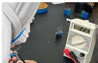
Gambar 9 Nilai kapasitor baru 220 \mu F
