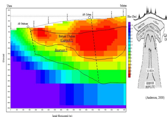
Gambar 6. Penampang resistivitas bawah permukaan
