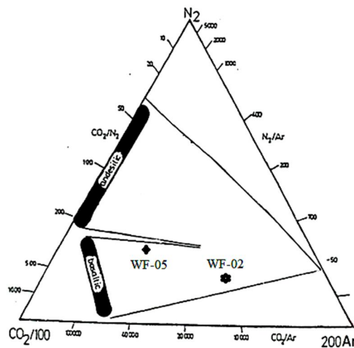
Gambar 5. Diagram ternary geointikator CO 2 /N 2 , N 2 /Ar dan CO 2 /Ar
