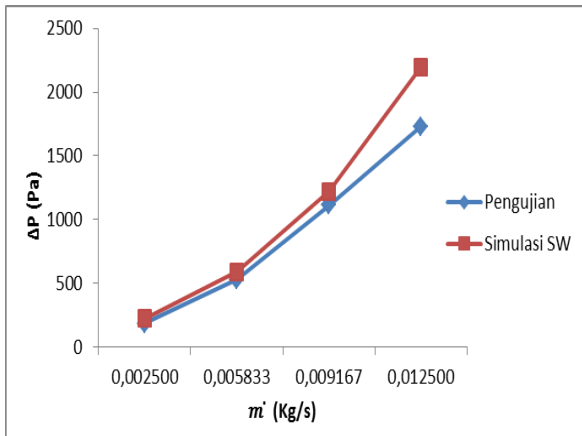
Gambar 8. Grafik pressure drope kolektor surya W 40 mm rangkaian vertical sambungan U-bend.
