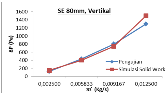
Gambar 3. Grafik pressure drope Kolektor surya W 80 mm rangkaian vertikal
