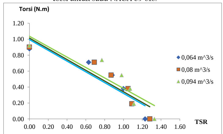
Gambar 12. Grafik hubungan tip speed ratio (TSR) terhadap torsi untuk sudu NREL S833.
