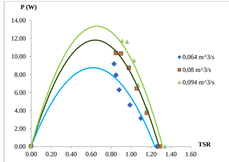
Gambar 14. Grafik hubungan tip speed ratio (TSR) terhadap daya poros sudu NACA 63-818.
