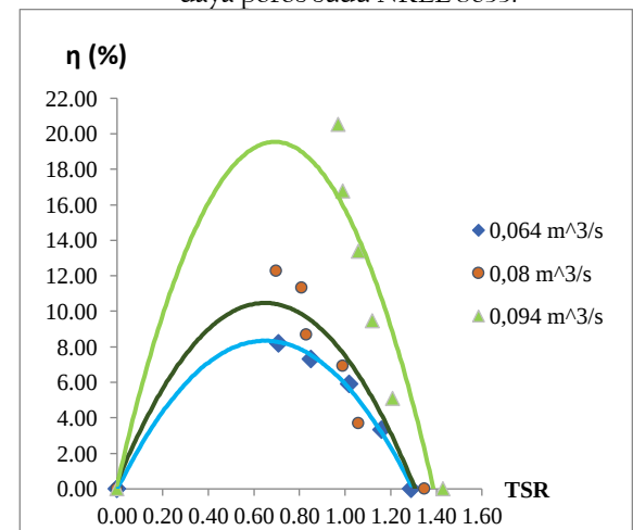
Gambar 16. Grafik hubungan tip speed ratio (TSR) terhadap efisiensi sudu RISO A-18.
