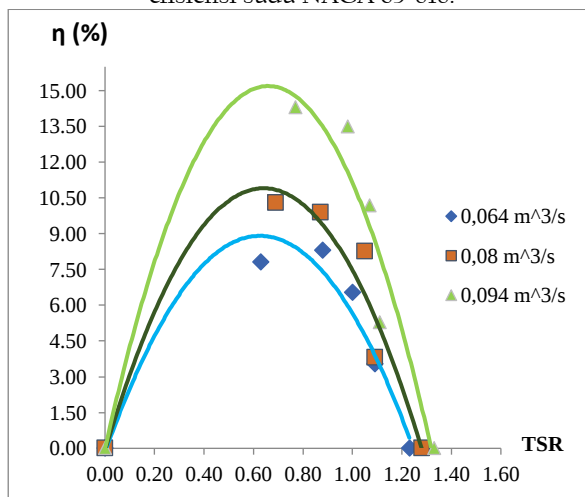
Gambar 18. Grafik hubungan tip speed ratio (TSR) terhadap efisiensi sudu NREL S833.
