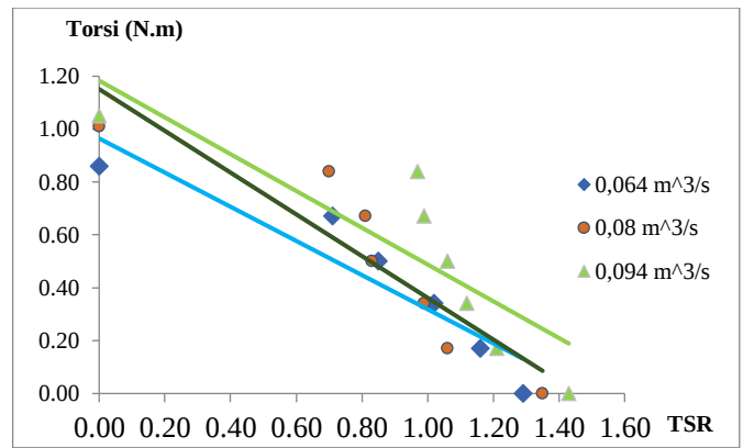
Gambar 10. Grafik hubungan tip speed ratio (TSR) terhadap torsi untuk sudu RISO A-18.
