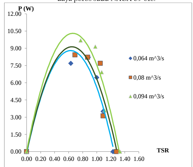
Gambar 15. Grafik hubungan tip speed ratio (TSR) terhadap daya poros sudu NREL S833.
