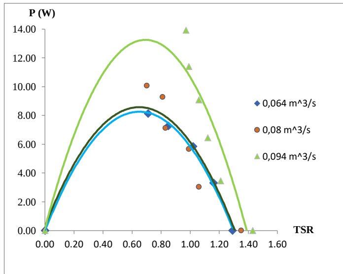
Gambar 13. Grafik hubungan tip speed ratio (TSR) terhadap daya poros sudu RISO A-18.
