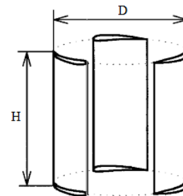
Gambar 1. Skema turbin Darrieus sudu lurus.
