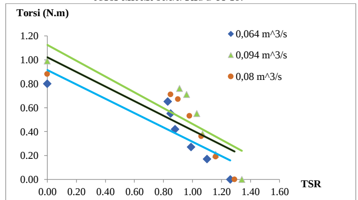
Gambar 11. Grafik hubungan tip speed ratio (TSR) terhadap torsi untuk sudu NACA 63-818.
