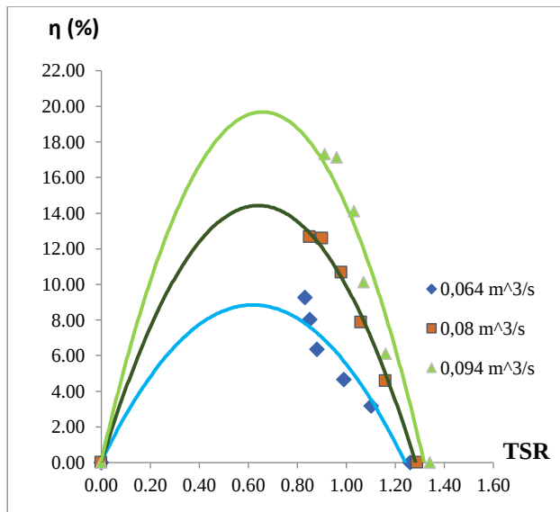
Gambar 17. Grafik hubungan tip speed ratio (TSR) terhadap efisiensi sudu NACA 63-818.
