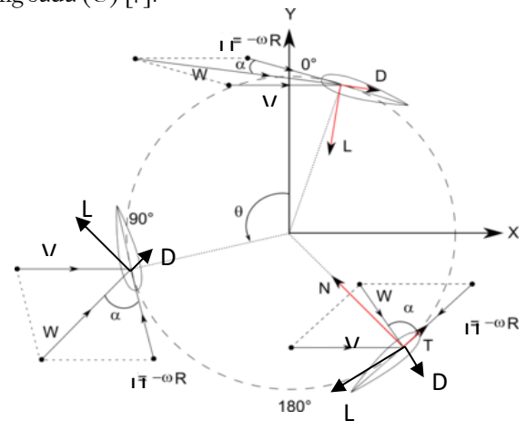
Gambar 4. Poligon kecepatan pada turbin sumbu vertikal
