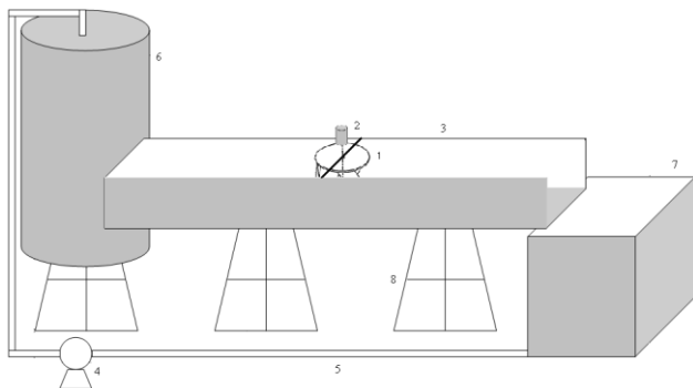
Gambar 4. Skema model alat pengujian.
