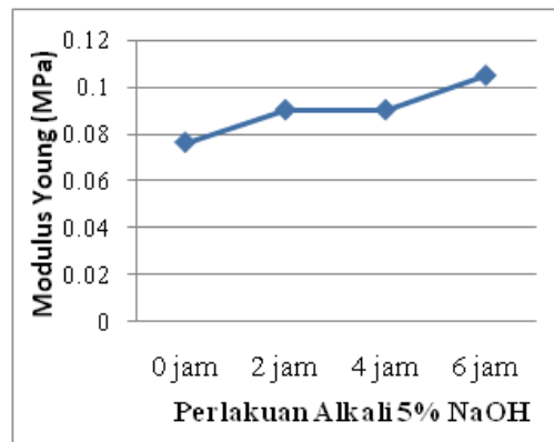
Gambar 8. Grafik hubungan Modulus Young dengan perlakuan alkali.
