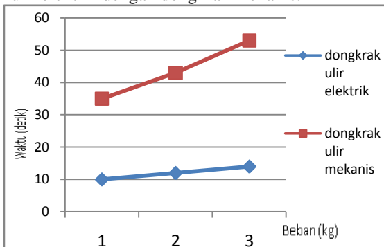
Gambar 6. Grafik perbandingan berat beban yang diangkat dengan waktu operasi pada dongkrak ulir elektrik dan dongkrak mekanis.
