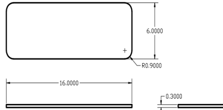
Gambar 4. Desain plat tambahan dudukan bagian bawah
