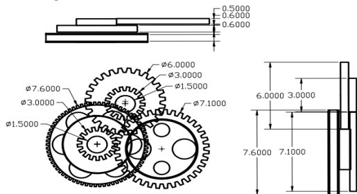
Gambar 2. Desain kedudukan gearbox dan motor.
