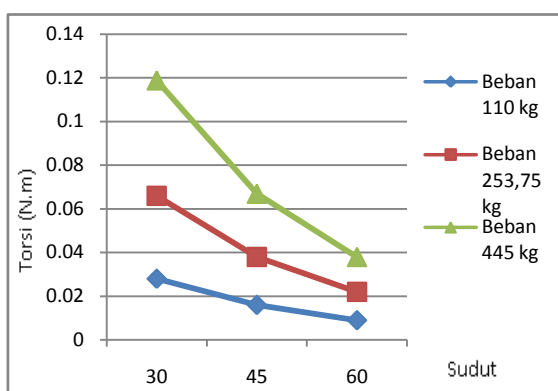
Gambar 8. Grafik perbandingan besar sudut dengan torsi inputan yang dibutuhkan gearbox untuk ditransmisikan pada dongkrak ulir.
