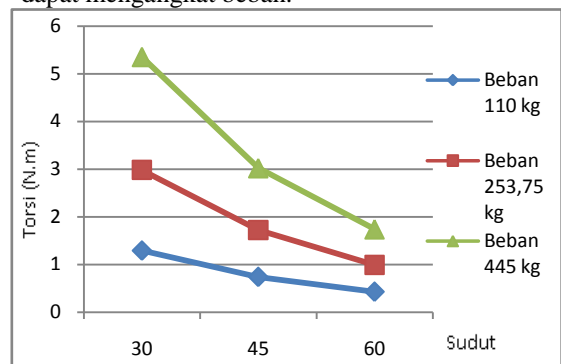
Gambar 7. Grafik perbandingan besar sudut dengan torsi inputan yang dibutuhkan dongkrak ulir.
