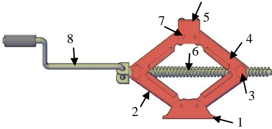
Gambar 1. Komponen-komponen dongkrak ulir mekanis Keterangan gambar:
