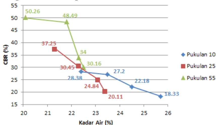
Gambar 3. Hubungan nilai CBR dengan Kadar Air
