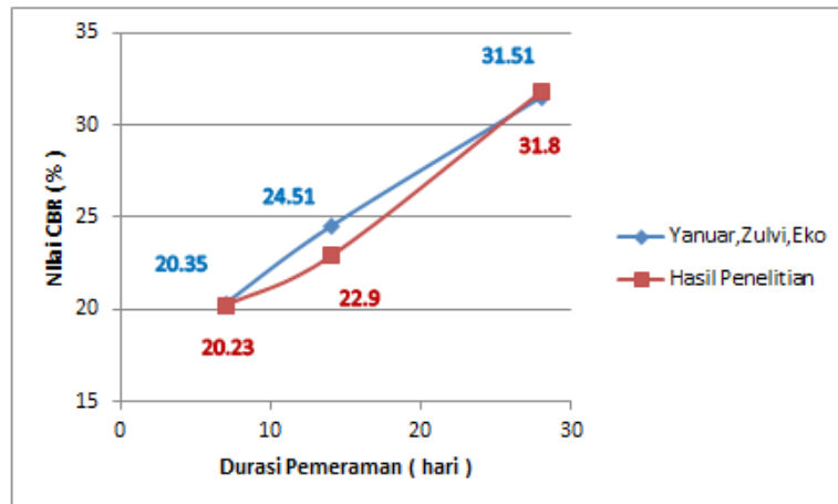
Gambar 5. Hubungan durasi pemeraman dengan nilai CBR
