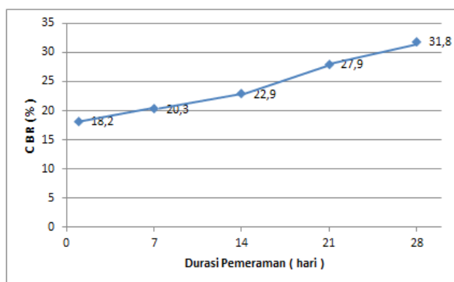
Gambar 1. Hubungan durasi pemeraman dengan nilai CBR
