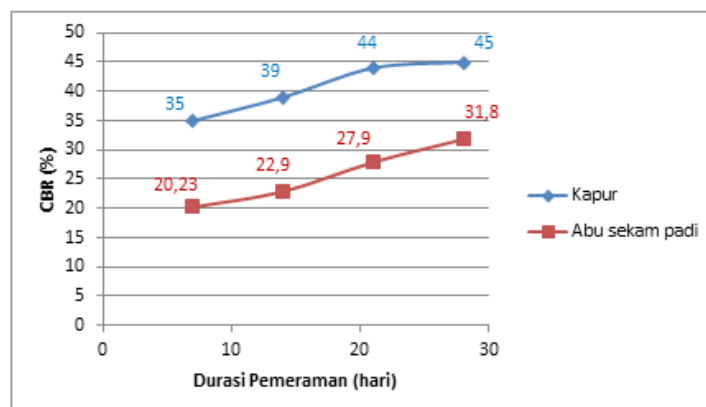
Gambar 6. Hubungan durasi pemeraman dengan nilai CBR
