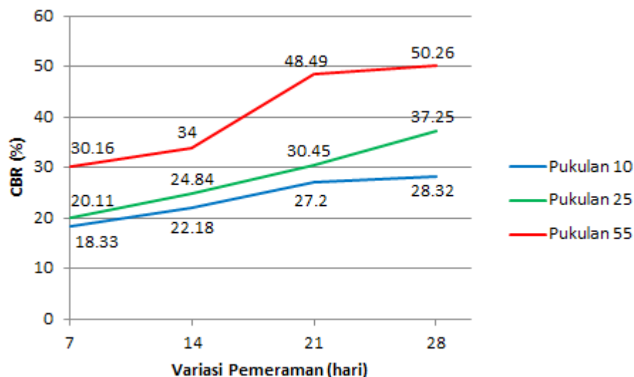
Gambar 2. Hubungan nilai CBR dengan Variasi Pukulan
