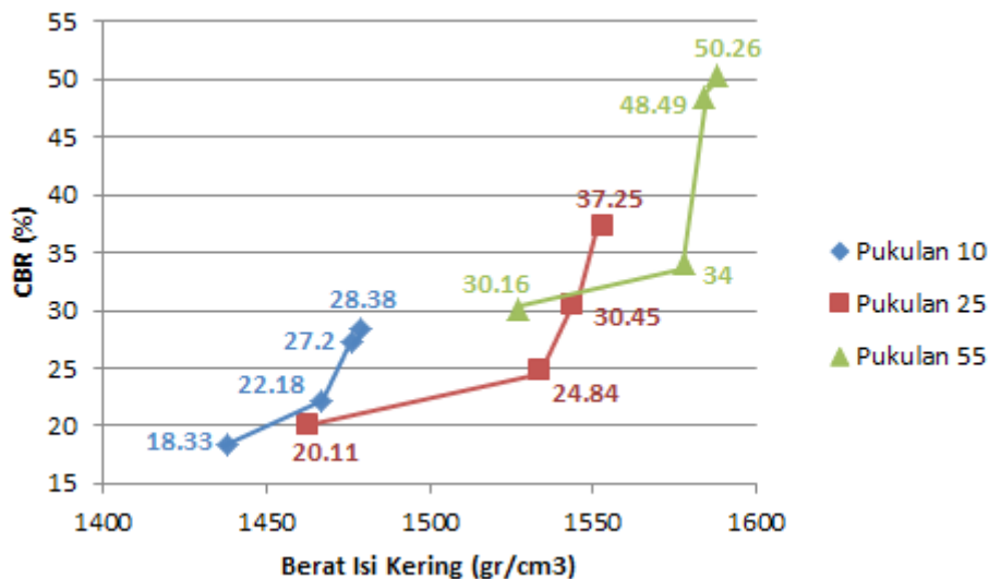
Gambar 4. Hubungan nilai CBR dengan Berat Isi Kering
