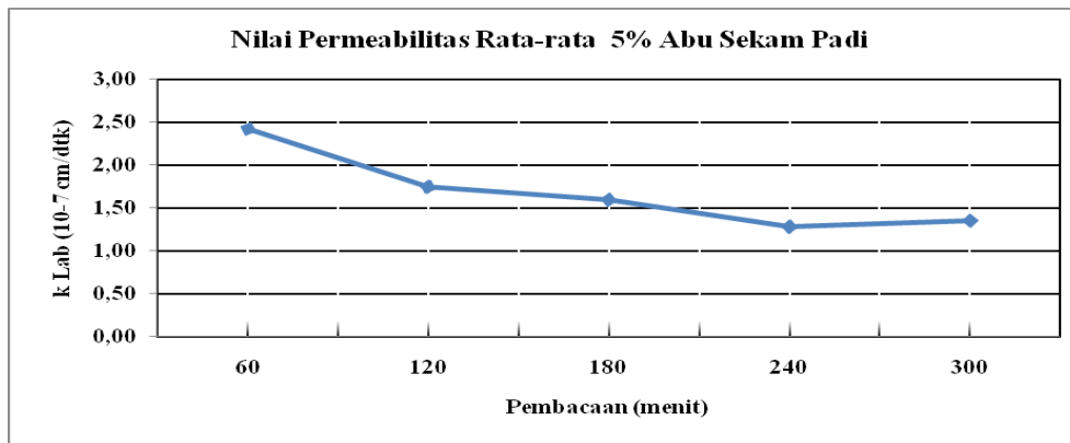
Gambar 3. Grafik Permeabilitas Campuran 5% Abu Sekam Padi.
