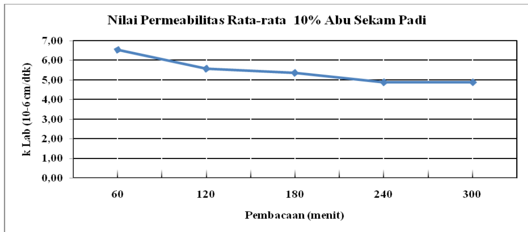
Gambar 4. Grafik Permeabilitas Campuran 10% Abu Sekam Padi.
