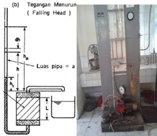
Gambar 1. Alat Uji Permeabilitas.
