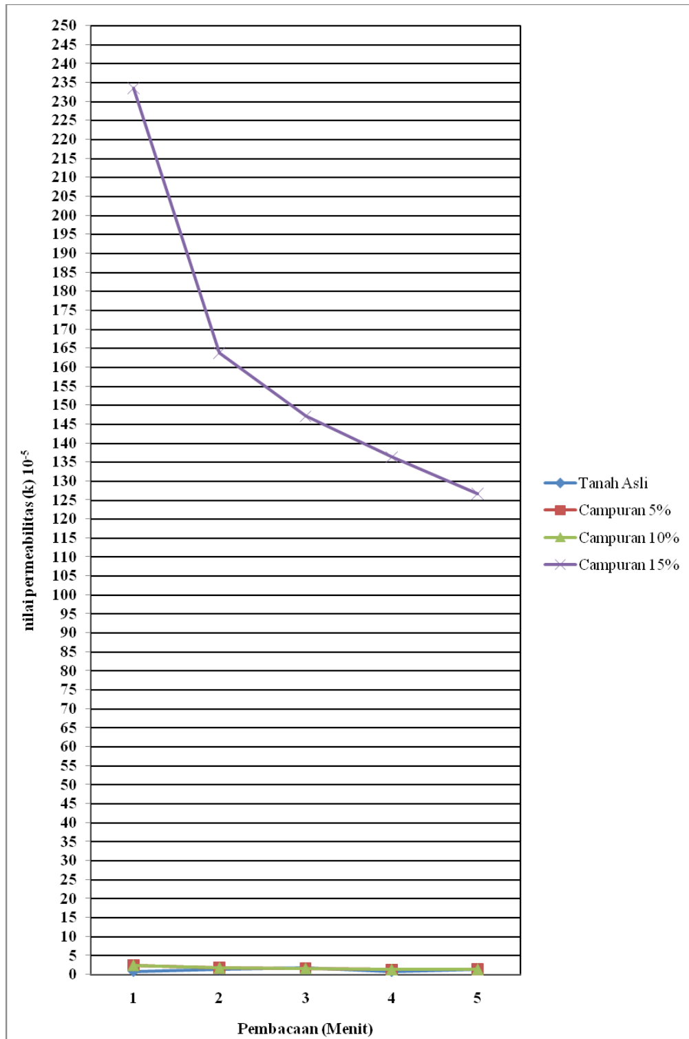
Gambar 6. Grafik Perbandingan Nilai Permeabilitas.
