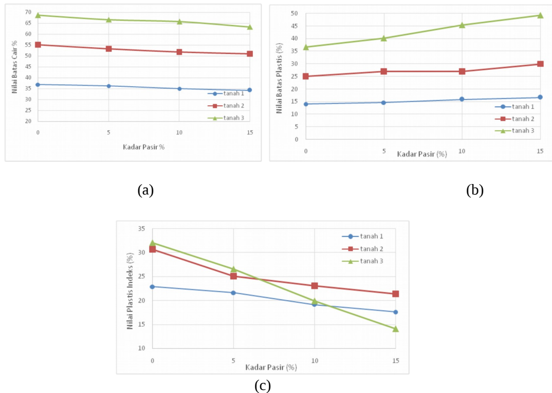
Gambar 3. (a). Hubungan Campuran Pasir dan Batas Cair (b). Hubungan Campuran Pasir dan Batas Plastis (c). Hubungan Campuran Pasir dan Plastisitas Indeks.
