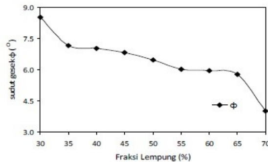
Gambar 2. Hasil uji Triaksial untuk sudut gesek
