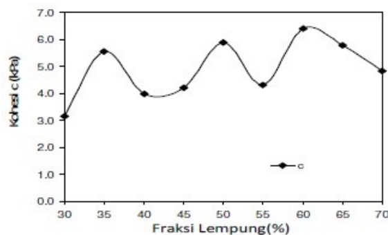
Gambar 3. Hasil uji Direct Shear untuk nilai kohesi
