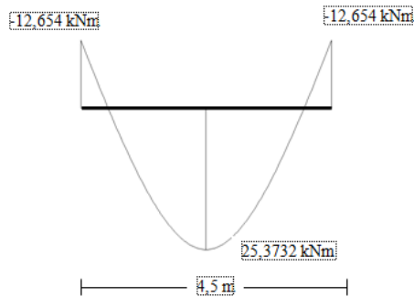
Gambar 5 Momen Lentur Pelat Melebar Metode Elemen Hingga
