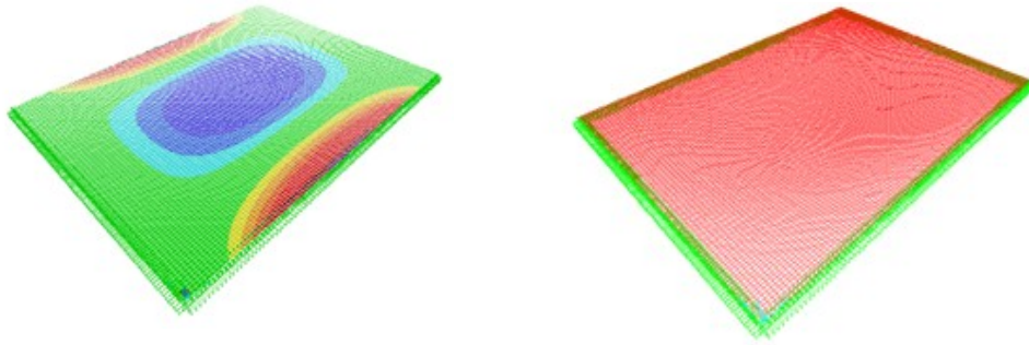
Gambar 3. Momen Lentur dan Lendutan Pelat Elemen Segiempat
