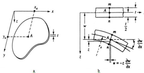
Gambar 1. (a) Pelat dengan Tebal Konstan; (b) Bagian dari Pelat Sebelum dan Sesudah Defleksi.
