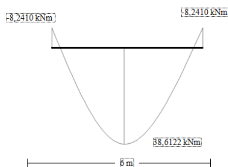
Gambar 4. Momen Lentur Pelat Memanjang Metode Elemen Hingga
