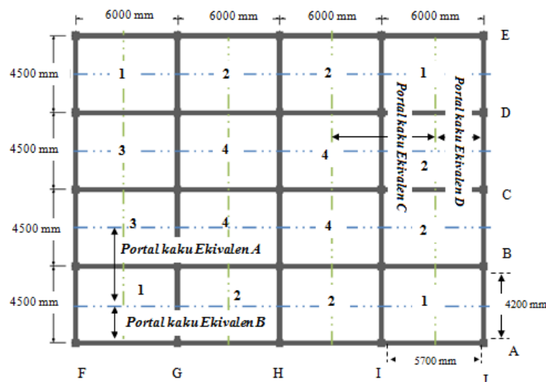
Gambar 2. Denah Pelat Lantai
