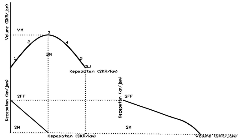
Gambar 1. Hubungan matematis antara volume, kecepatan, dan kepadatan.
