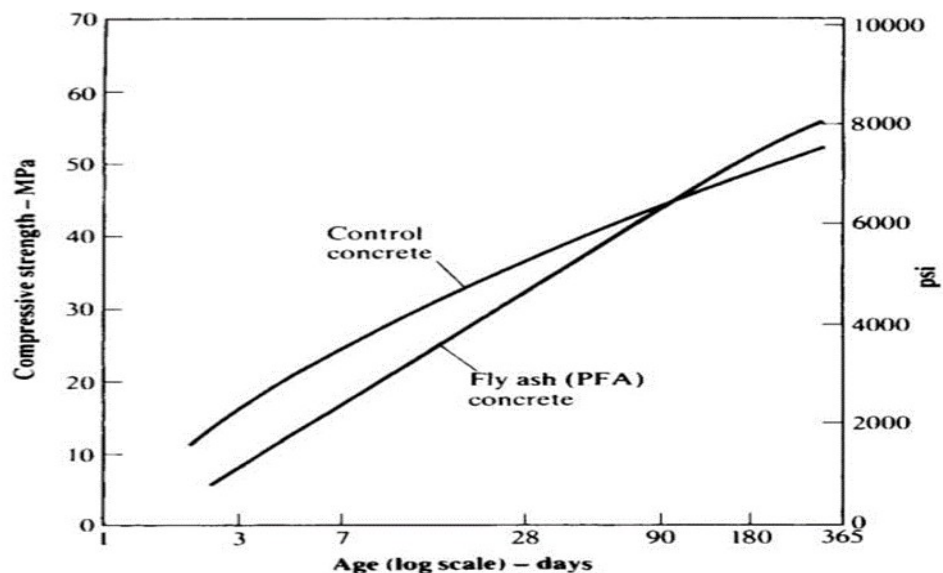
Gambar 8. Perbandingan kuat tekan beton terhadap umur beton.
