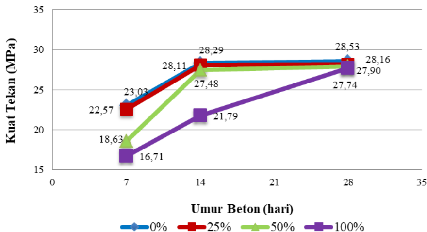
Gambar 5. Hubungan nilai kuat tekan beton terhadap faktor umur beton
