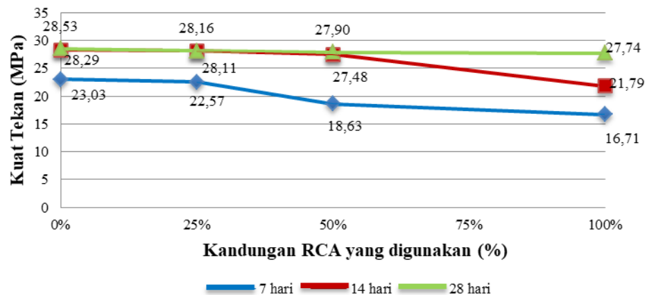
Gambar 4. Hubungan nilai kuat tekan beton dengan variasi penggantian sebagian agregat kasar dengan RCA
