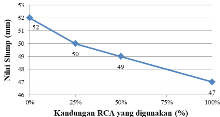
Gambar 2. Hubungan antara nilai slump dengan variasi penggantian sebagian Agregat kasar dengan RCA.
