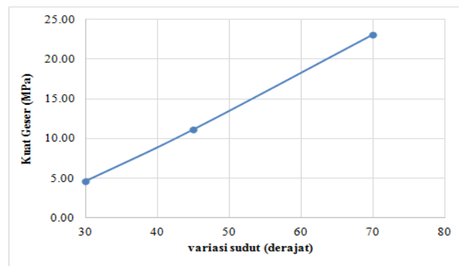
Gambar 3. Grafik kuat geser interface variasi sudut.
