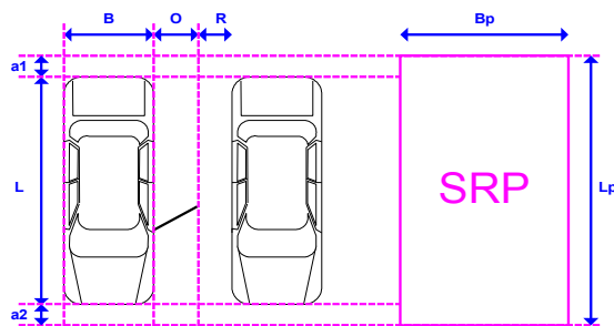
Gambar 1. Satuan Ruang Parkir Untuk Mobil Penumpang
