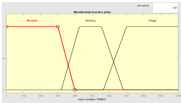
Gambar 3.5 Fungsi Keanggotaan Sensor Debu GP2Y
