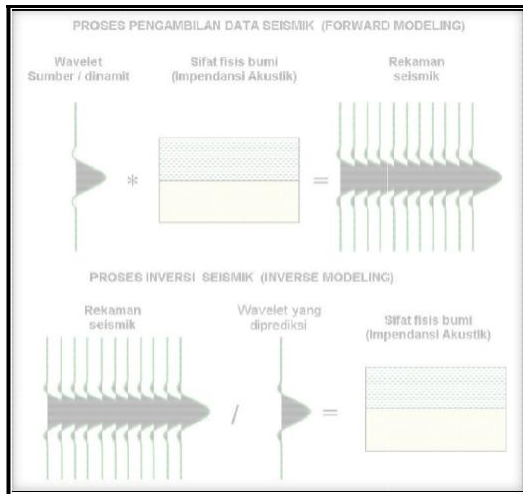
Gambar 2. konsep dasar inversi seismik (Abdullah, 2008).
