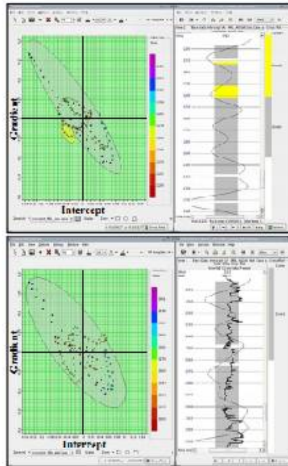
Gambar 7. Analisis crossplot antara Intercept dan gradient pada sumur Vanda-2 (atas) Gas Case , (bawah) Wet Case
