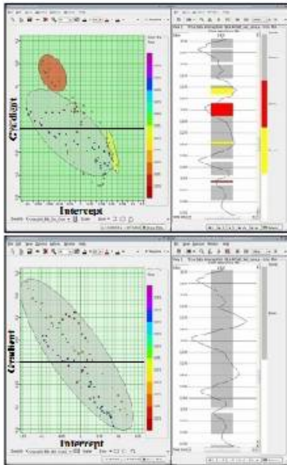
Gambar 6. Analisis crossplot antara Intercept dan gradient pada sumur Vanda-1 (atas) Gas Case , (bawah) Wet case
