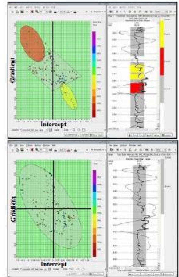
Gambar 8. Analisis crossplot antara Intercept dan gradient pada sumur Vanda-3 (atas) Gas Case , (bawah) Wet Case .
