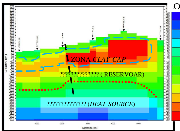
Gambar 7. Model 2D tahanan jenis line 1 Setelah pendekatan inversi 1D
