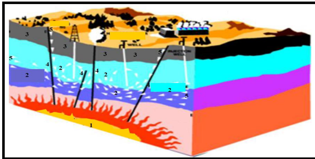
Gambar 1. Model sistem panas bumi secara umum (dimodifikasi dari geothermal figure google 18 Agustus 2010), (1) sumber panas, (2) reservoir, (3) lapisan penutup, (4) patahan, (5) daerah resapan ( recharge area ) (google geothermal , 2010).
