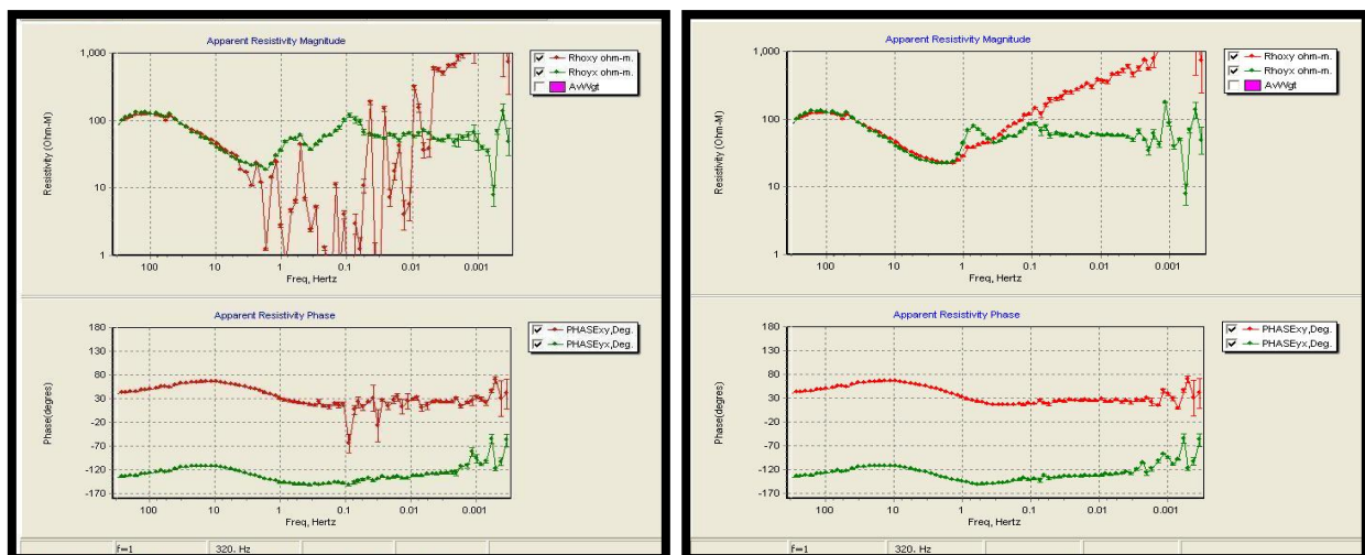
Gambar 3. Kurva apparent resistivity belum diedit (Kiri) dan sudah di edit (Kanan)
