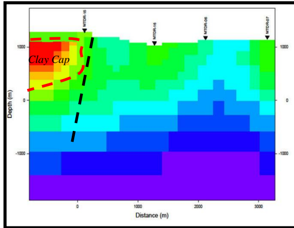
Gambar 9. Model tahanan jenis setelah di analisis inversi 1D.
