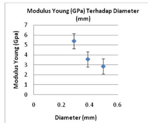
Gambar 13. Grafik deviasi modulus elastisitas Terhadap Diameter Serat Ijuk
